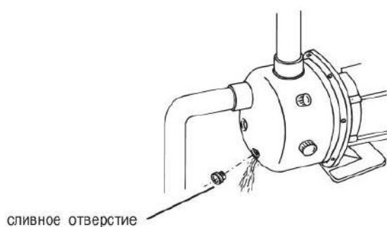
Рис. 7 Осушение рабочей полости насоса
