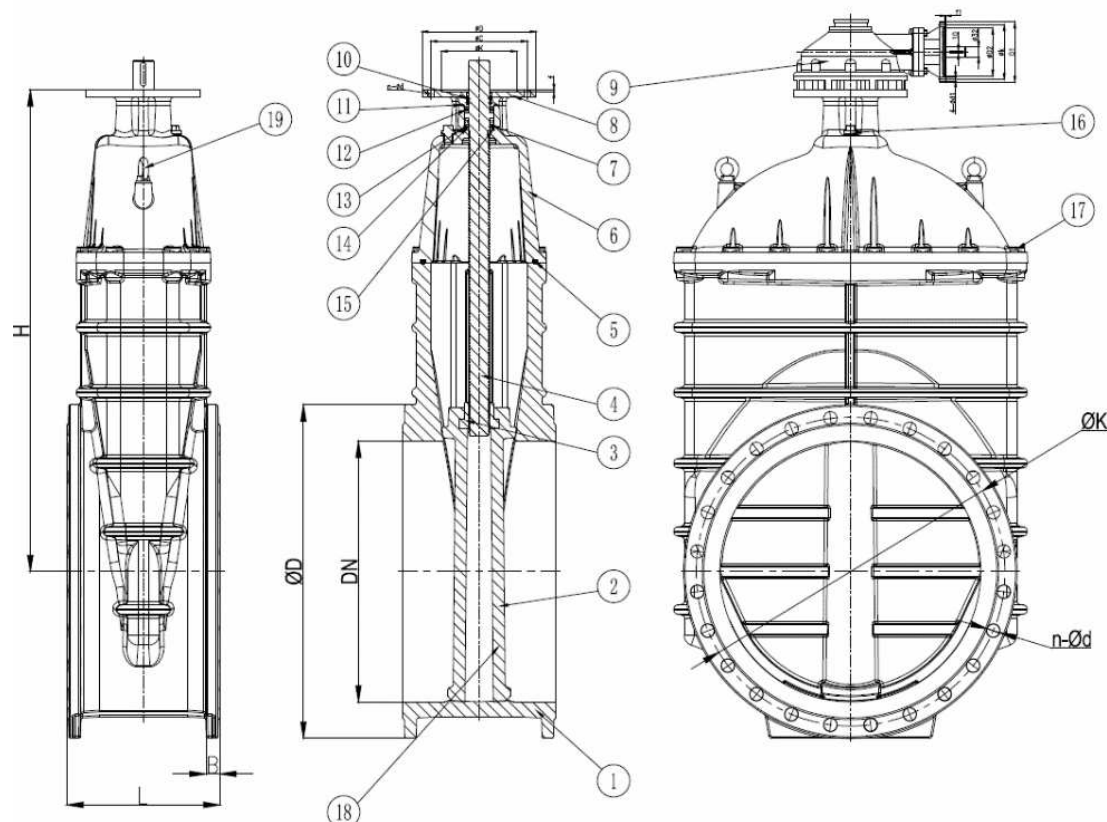
Рис. 1. Задвижка чугунная 30ч539р фланцевая с редуктором.
