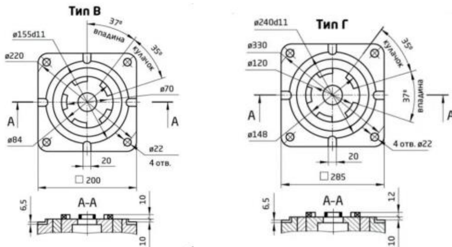
Рис.2. Присоединительные размеры верхнего фланца (ОСТ) задвижки 30с941нж под электропривод.
