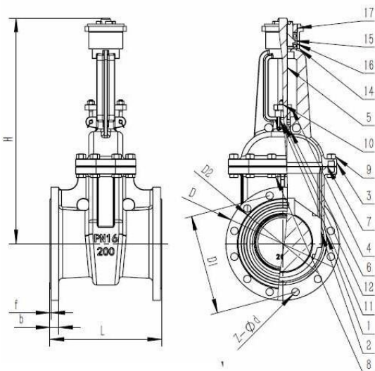
Рис.2. Задвижка 30с941нж Ду200-Ду300
